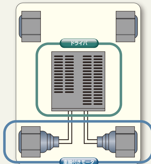
AGV の構成イメージ
