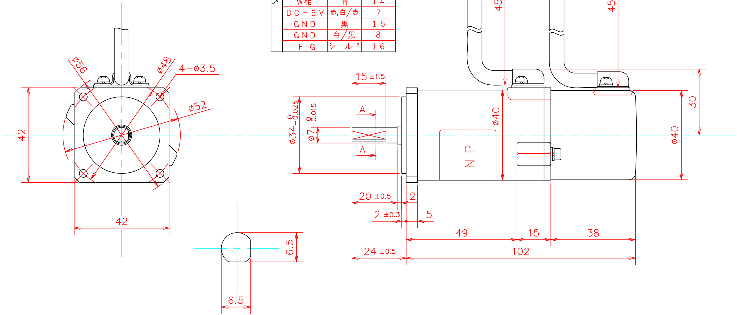
A-A断面 (S=2/1)
